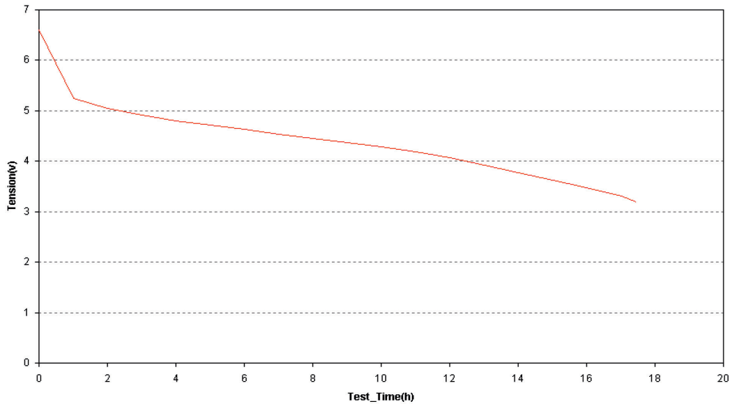
Decharge sur 4.7ohms
